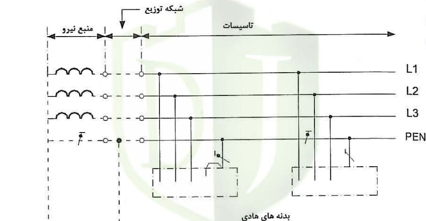
اتصال زمین حفاظتی در شبکه توزیع اتصال زمین سیستم نیرو سیستم اتصال زمین با یک و یا چند الکترود زمین
