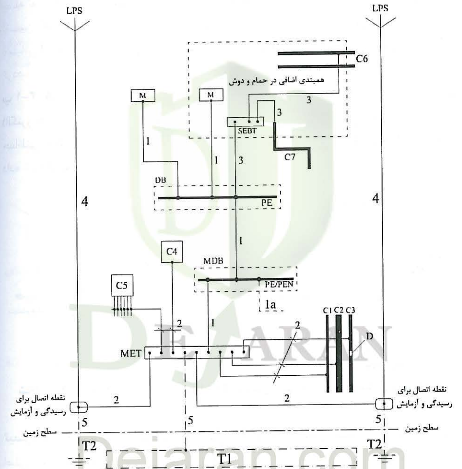
شکل پ ۴-۸-۲-۱ طرحواره عمومی همبندی اصلی و اضافی برای هم‌ولتاژ کردن
