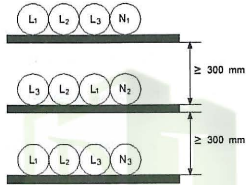
شکل ۱۳-۷-۱-۷-۱:۵ آرایش چسبیده به هم در سه تراز و هر تراز به فاصله ۳۰ سانتی متر از هم برای ۹ رشته کابل تکررشته موازی (سه فاز)
