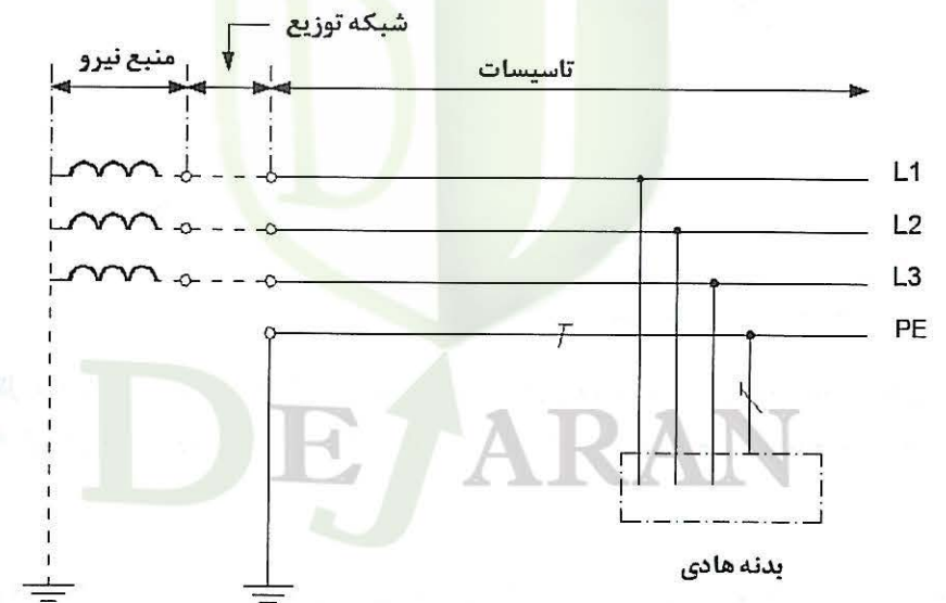
شکل پ ۱-۱:۵ سیستم TT در سیستم سه فاز با هادی حفاظتی و بدون توزیع هادی خنثی در سرتاسر سیستم
