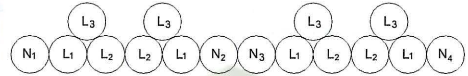
شکل ۷-۱۳-۱-۷-۱۳ آرایش مثلثی کنار هم برای ۱۲ رشته کابل تک‌رشته موازی (سه فاز)
