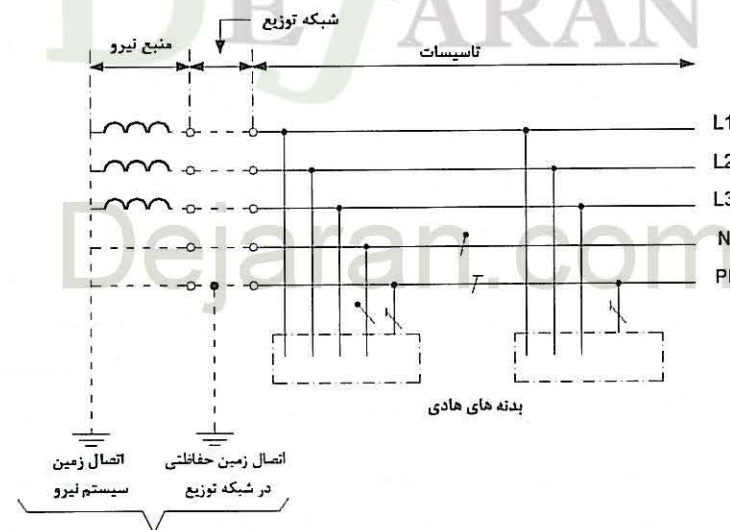
سیستم اتصال زمین با یک و یا چند الکترود زمین
