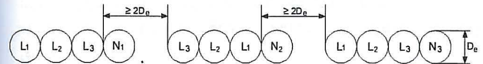
شکل ۱۳-۷-۱-۷-۱:۴ آرایش مخصوص همتراز برای ۹ رشته کابل تکررشته موازی (سه فاز)
