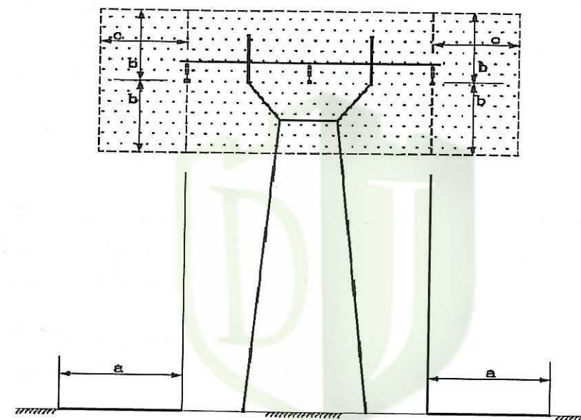
شکل پ ۷-۲-۲: خط هوایی فشار قوی (۶۳ کیلوولت و بالاتر)
