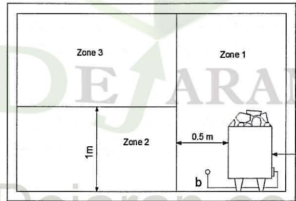
دید از کنار b = جعبه اتصال مدار تغذیه گرمکن برقی سونا
