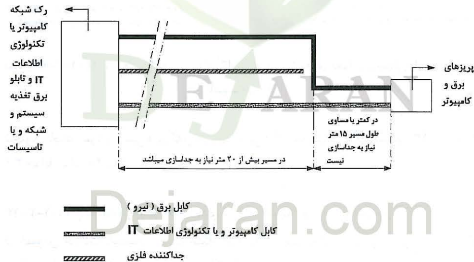
شکل ۱۳-۳-۲: ۲:۱-۱۸-۱-۳-۱۳ طرحواره مسیر مجزا و مشترک کابل برق و کابل کامپیوتر یا فناوری اطلاعات IT برای طول مسیر بیش از ۳۵ متر
