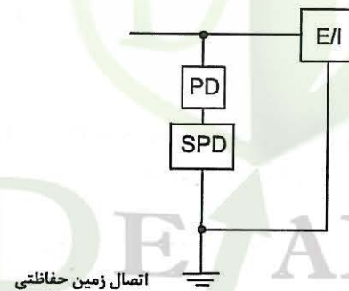
شکل ۱۳-۱-۳-۱۶-۳ طرحواره نصب وسیله حفاظتی و برقگیر حفاظتی در تابلو برق تغذیه‌کننده دستگاه و یا تجهیزات
