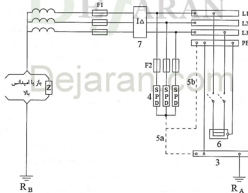
شکل ۳-۱۳-۱۶-۴: طرحواره نصب برقگیر حفاظتی در شبکه توزیع سیستم نیروی IT
