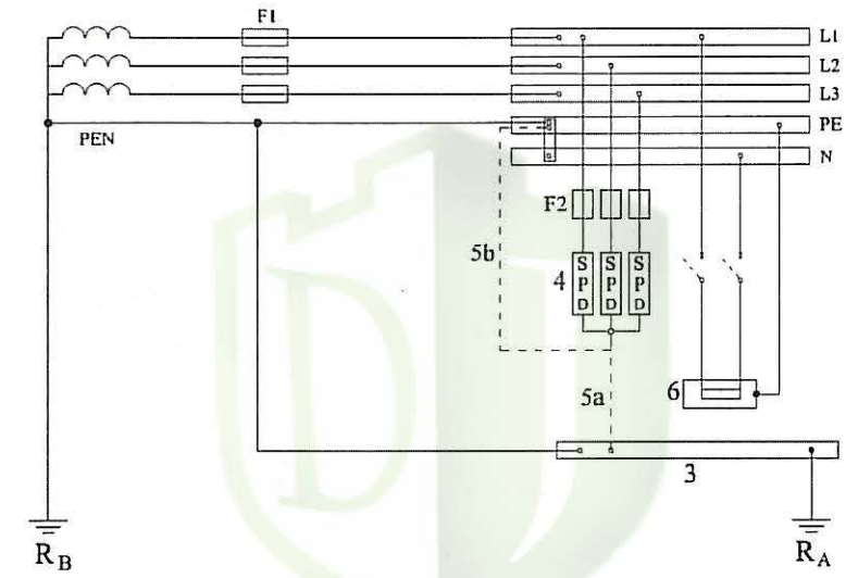
شکل ۳-۱۳-۱۶-۱: طرحواره نصب برقگیر حفاظتی در شبکه توزیع سیستم نیروی TN (سه فاز)
