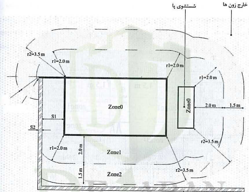
شکل ۱۰-۱۳-۵:۳-۴: طرح حواره ابعاد مناطق (zone) استخر، با دیوار جداکننده ثابت حداقل به ارتفاع ۲/۵ متر (دید از بالا)
