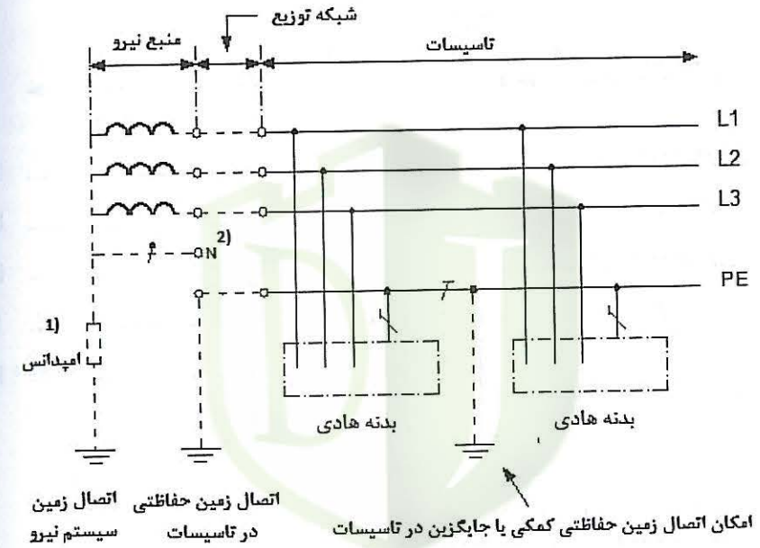
شکل پ ۱-۱-۷ سیستم IT که در آن کلیه بدنه‌های هادی به صورت گروهی از طریق یک هادی حفاظتی به اتصال زمین حفاظتی وصل گردیده است.
