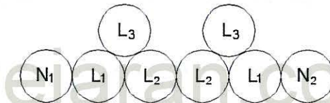
شکل ۱۳-۷-۱-۷-۱:۳ آرایش مثلثی چسبیده به هم برای ۶ رشته کابل تکررشته موازی (سه فاز)
