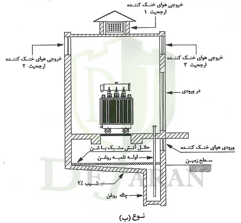
شکل ۱۳-۵-۳-۱ (نوع ب) - طرحواره قائم اتاق ترانسفورماتور روغنی با تهویه طبیعی و بالاتر از سطح زمین
