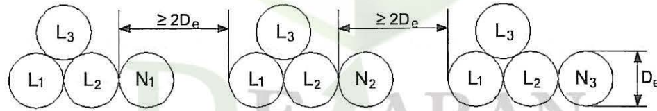
شکل ۱۳-۷-۱-۷-۱:۶ آرایش مثلثی مخصوص برای ۹ رشته کابل تکررشته موازی (سه فاز)
