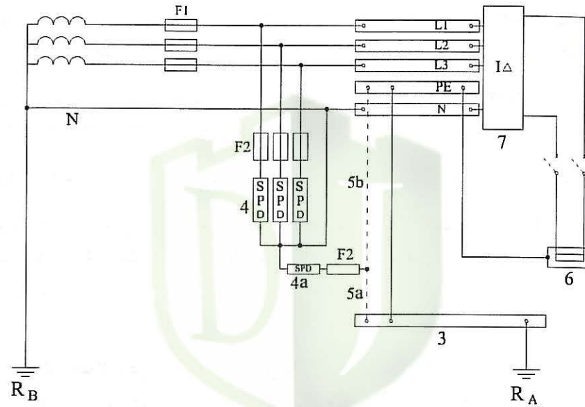
شکل ۳-۱۳-۱۶-۴: طرحواره نصب برقگیر حفاظتی در شبکه توزیع سیستم نیروی TT با قرارگیری برقگیر حفاظتی قبل از کلید حفاظتی جریان باقی مانده (RCD)
