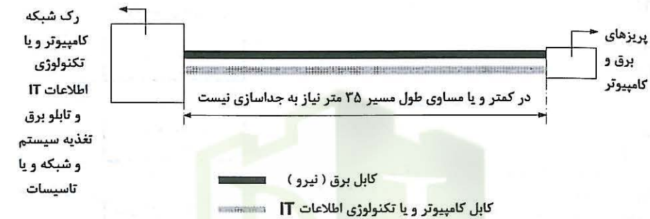
شکل ۱۳-۳-۱: ۱:۱-۱۸-۱-۳-۱۳ طرحواره مسیر مشترک کابل برق و کابل کامپیوتر یا فناوری اطلاعات IT برای طول مسیر کمتر یا مساوی ۳۵ متر
