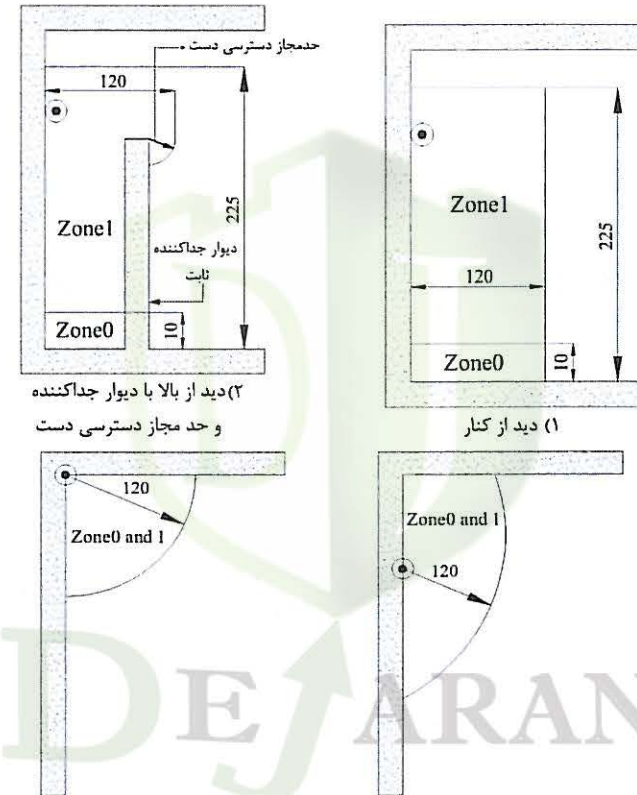
(۳) دید از بالا برای موقعیت‌های مختلف نصب دوش
