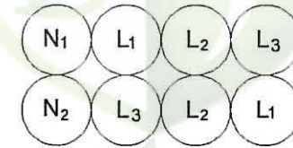
شکل ۱۳-۷-۱-۷-۱:۲ آرایش چسبیده به هم و در دو تراز برای ۶ رشته کابل تکررشته موازی (سه فاز)
