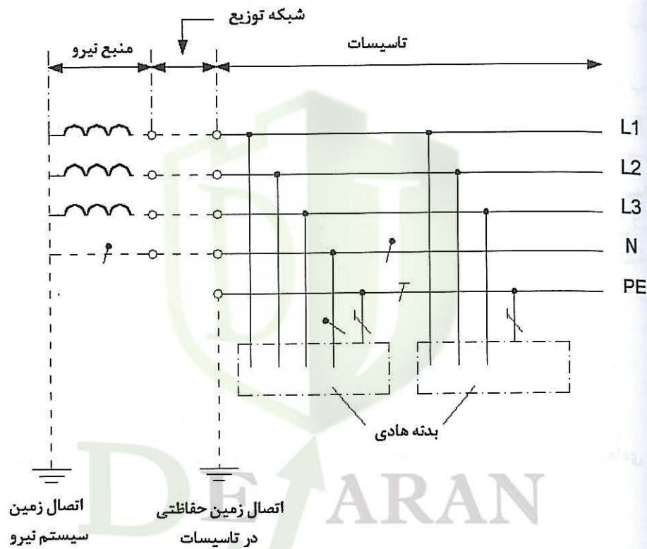
شکل پ ۱-۱:۶ سیستم TT در سیستم سه فاز با هادی حفاظتی و با توزیع هادی خنثی در سرتاسر سیستم
