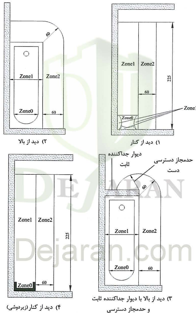
شکل ۱۳-۴-۱:۲ طرحواره موقعیت و ابعاد مناطق (zone) ها یا موقعیت زیردوش
