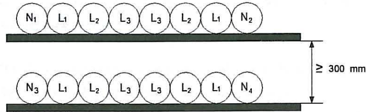
شکل ۱۳-۷-۱-۷-۱:۸ آرایش چسبیده به هم در دو تراز به فاصله ۳۰ سانتی متر از هم برای ۱۲ رشته کابل تکررشته موازی (سه فاز)
