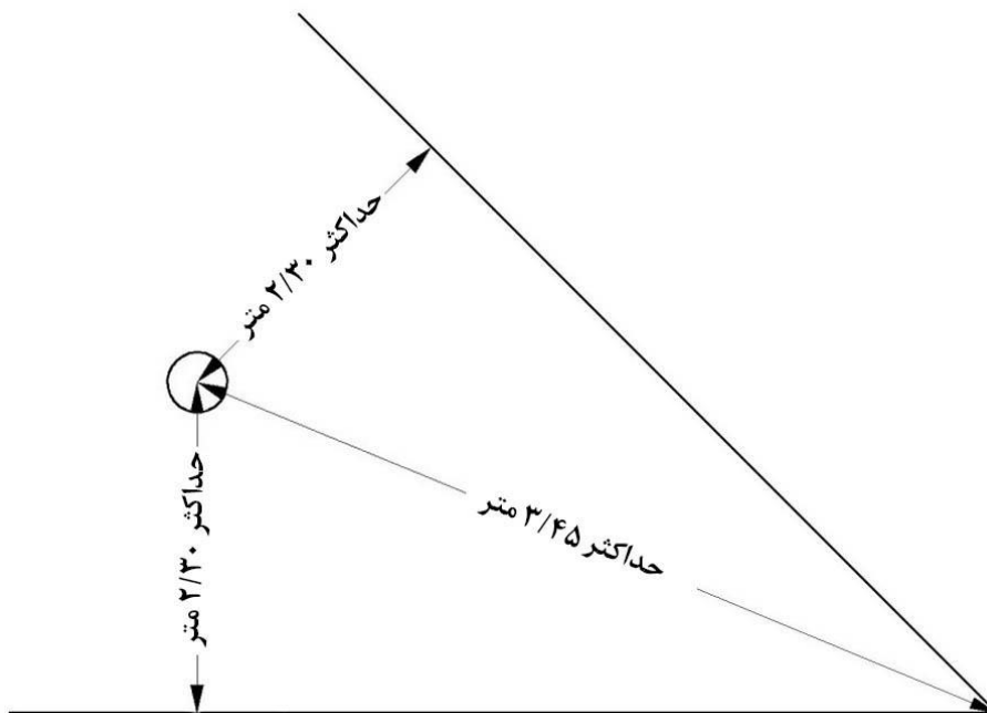
شکل ۱۱-۴-۴- حداکثر فاصله اسپرینکلر از کنج دیوار
