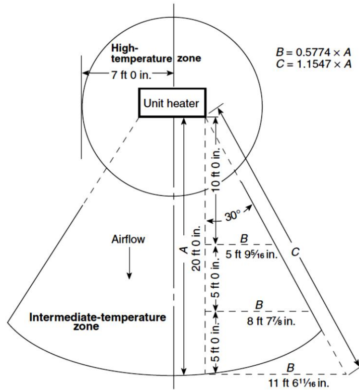
شکل ۴-۴-۷- مناطق دمابالا و دما متوسط در واحد حرارتی
