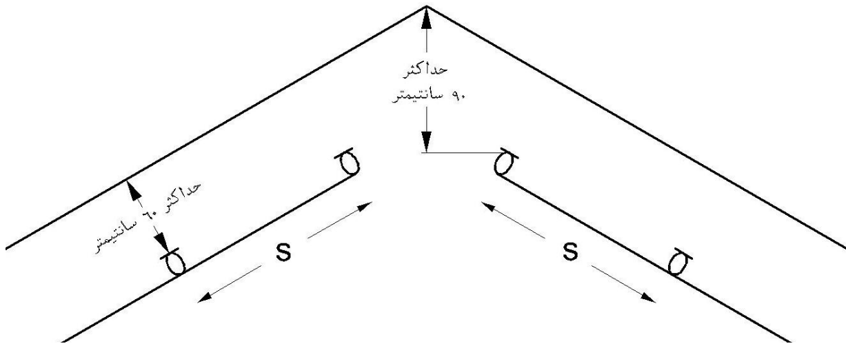
شکل ۴-۵-۱۵- نصب اسپرینکلر سقف‌های شیب‌دار
