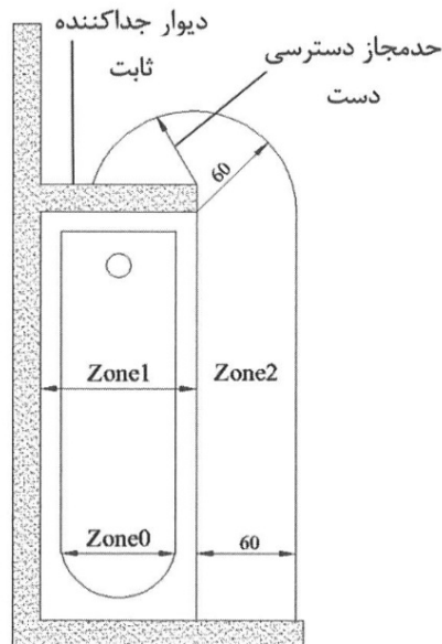
(۳) دید از بالا با دیوار جداکننده ثابت و دستمجاز دسترسی
