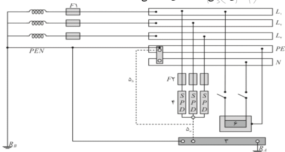
شکل طرحواره نصب برقگیر حفاظتی در شبکه توزیع سیستم نیروی TN (سه فاز)
